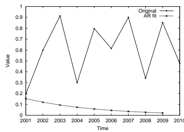
(d) The AR(1) fit
